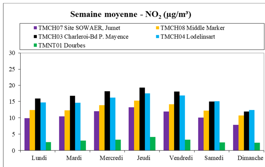
Figure 6.5.3 : Dioxyde d'azote (NO 2 ) – Semaine moyenne – (01/01/2024 au 31/12/2024)
