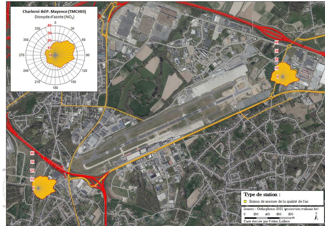
Figure 6.5.4 : Dioxyde d'azote (NO 2 ) – Roses de pollution – (01/01/2024 au 31/12/2024)
