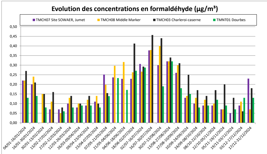
Figure 9.3.1 : Formaldéhyde ( \text{CH}_2\text{O} ) – Evolution des concentrations bimensuelles – (04/01/2024 au 31/12/2024)
