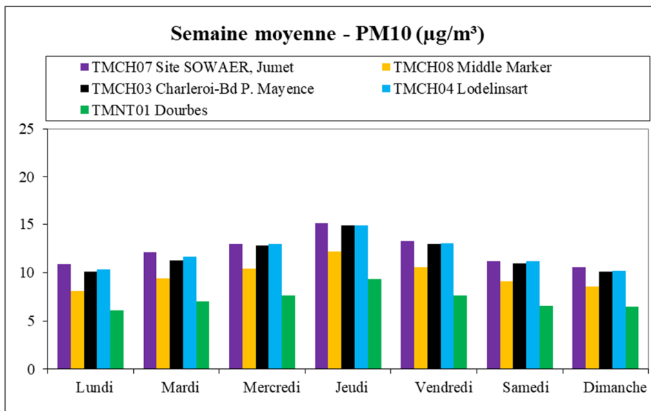
Figure 4.3.3 : PM10 – Semaine moyenne – (01/01/2024 au 31/12/2024)
