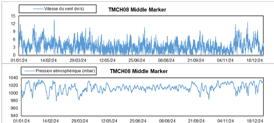
Figure 3.1 : Paramètres météorologiques – Evolution des valeurs semi-horaires – (01/01/2024 au 31/12/2024)
