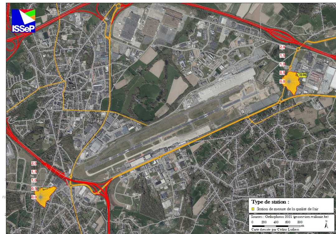
Figure 7.3.3 : Toluène ( C_6H_5-CH_3 ) – Roses de pollution – (01/01/2024 au 31/12/2024)
