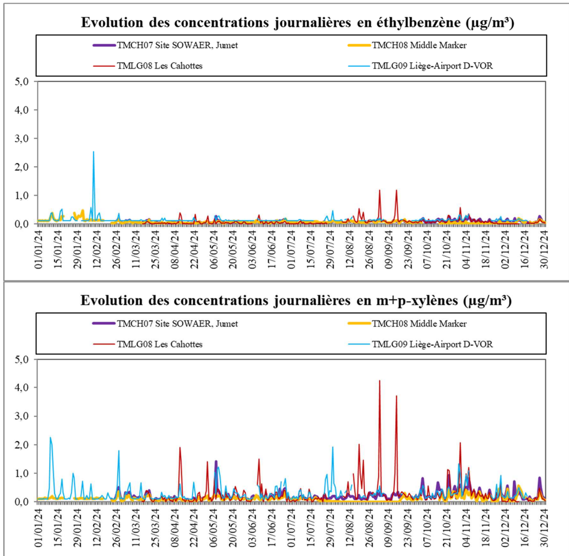
Figure 7.3.1 : BTEX – Evolution des concentrations journalières – (01/01/2024 au 31/12/2024)
