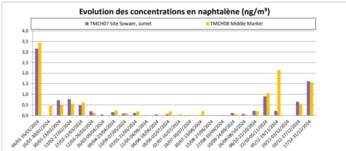
Figure 8.3.1 : Naphtalène (C 10 H 8 ) – Evolution des concentrations – (04/01/2024 au 31/12/2024)
