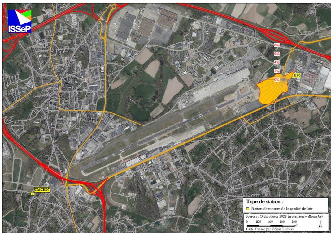
Figure 3.2 : Rose des vents – (01/01/2024 au 31/12/2024)
