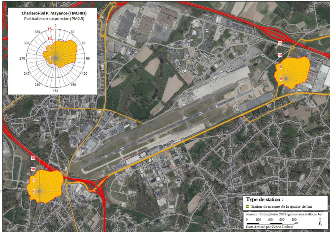
Figure 4.5.4 : PM2.5 – Roses de pollution – (01/01/2024 au 31/12/2024)
