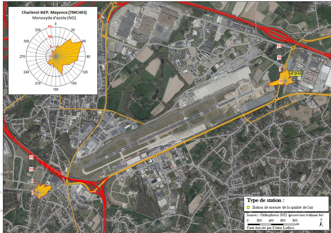
Figure 6.3.4 : Monoxyde d'azote (NO) – Roses de pollution – (01/01/2024 au 31/12/2024)
