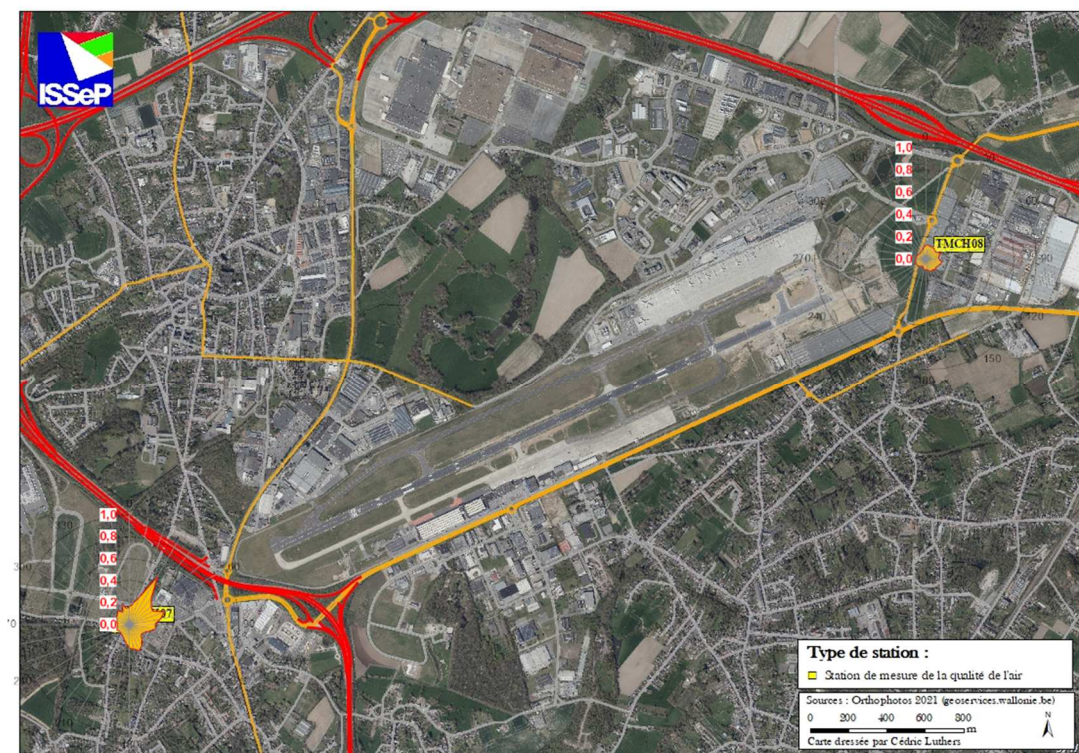
Figure 7.3.5 : m+p-xylènes ( C_8H_{10} ) – Roses de pollution – (01/01/2024 au 31/12/2024)
